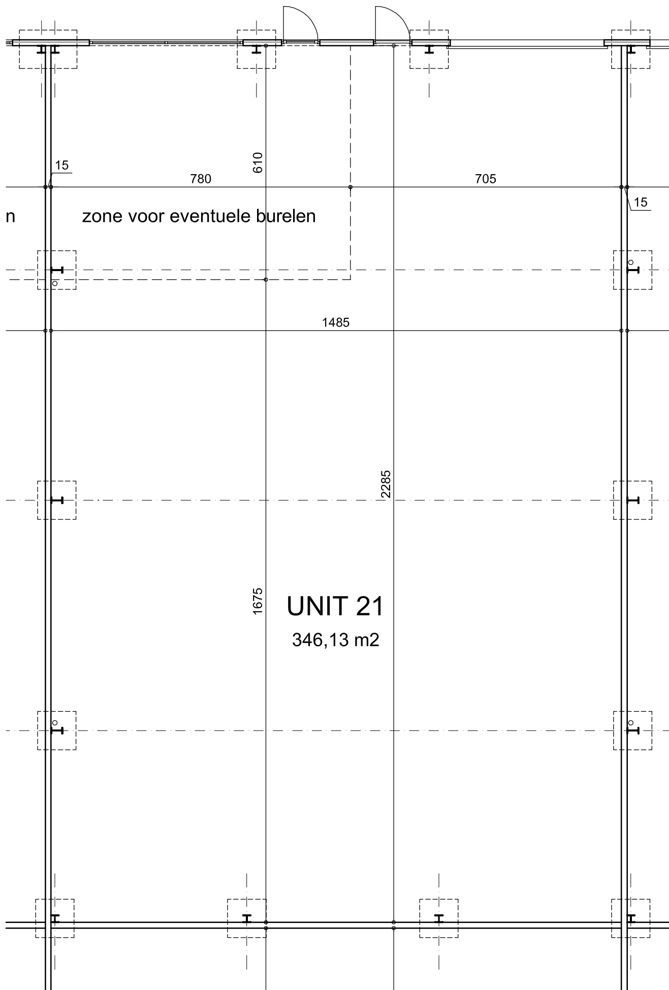
Grondplan schaal 1/100
